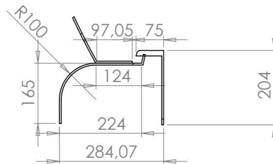
SZCZEGÓŁ B SKALA 1 : 10
